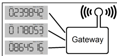
Abbildung 4: Beispielhaftes intelligentes Messsystem bestehend aus drei Basiszählern und einem Gateway.
