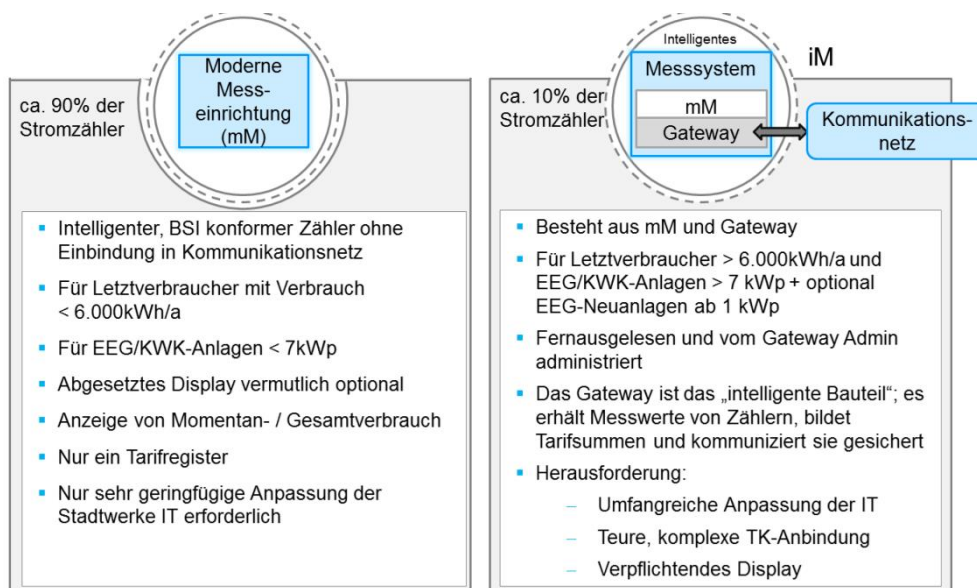
Abbildung 1: Übersicht moderne Messeinrichtung & intelligentes Messsystem
